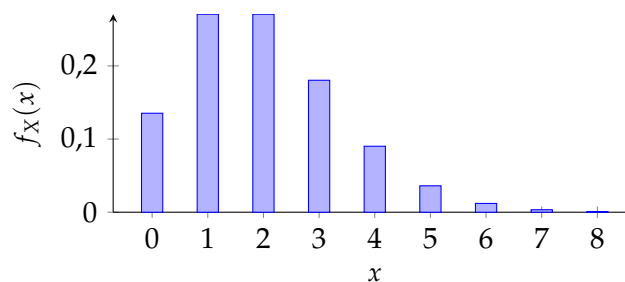
Poisson(2): el pico está cerca de \lambda = 2
